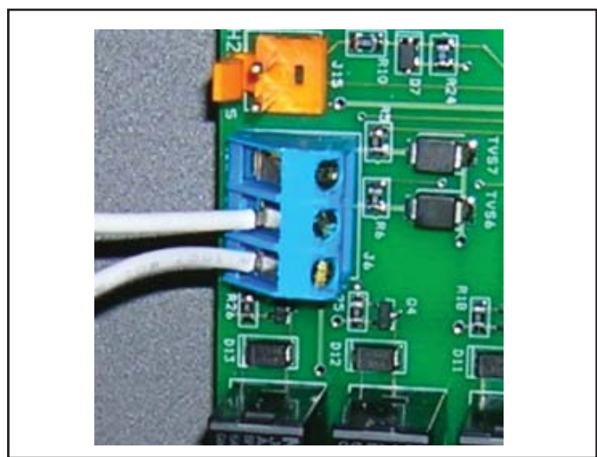
Figure 16b. Connexion de AquaLink RS ou de TSTAT à distance (Connexion bifilaire)
