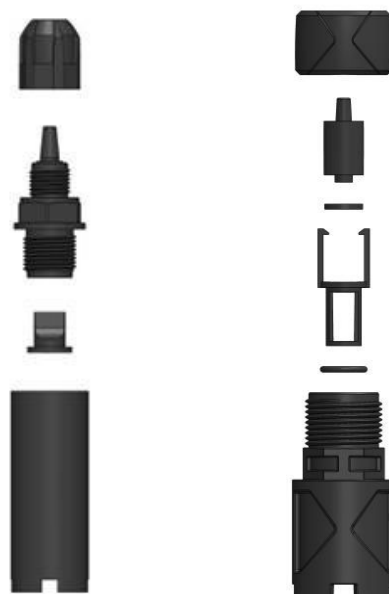
Vista despiezada
