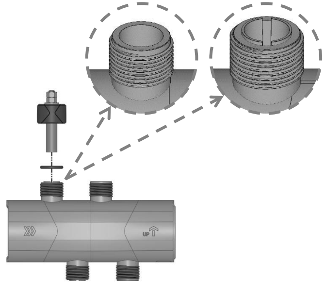
Sonda (pH u ORP) con portasonda
