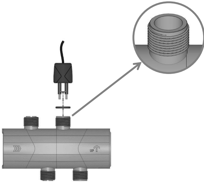
Insput-aansluitstuk met halfstijve slang
