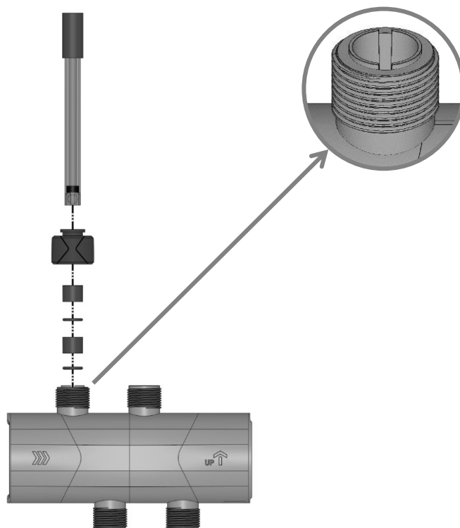
Sonda (pH ou ORP) com suporte para sondas
