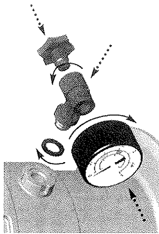
Montage du manomètre (sans vanne Top)
