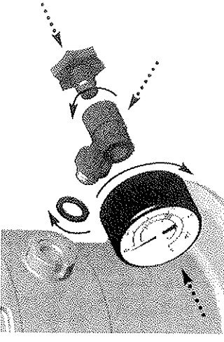
Montage du manomètre (sans vanne Top)
