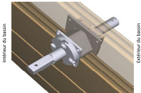
Figure 37 – Montage de l'arbre de couverture automatique
