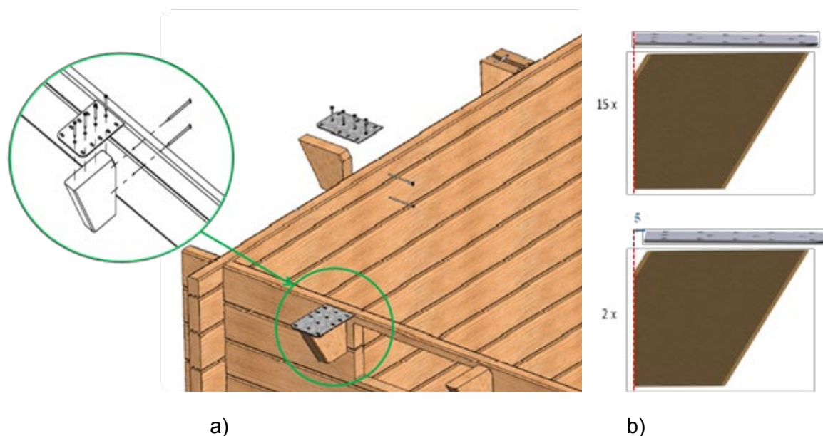
Figure 13 – a et b - Montage des plaques métalliques sur les consoles de margelles
