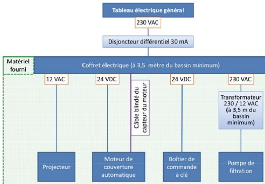
Figure 52 – Schéma électrique de principe de la PISCINE URBAINE
