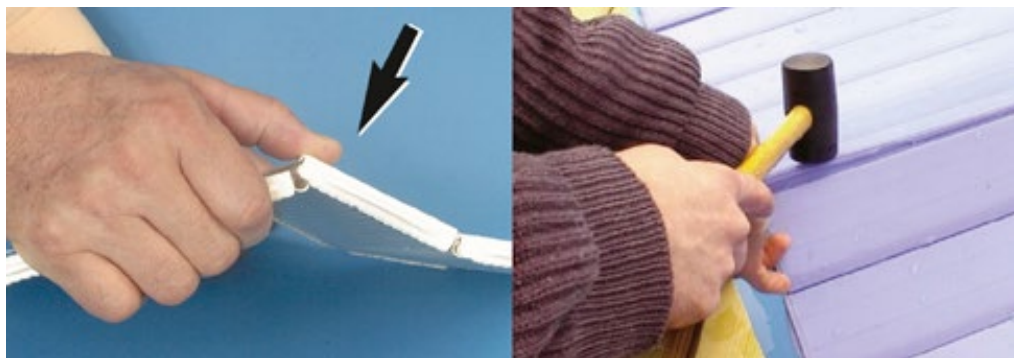
Figure 43 – Clipsage des lames
