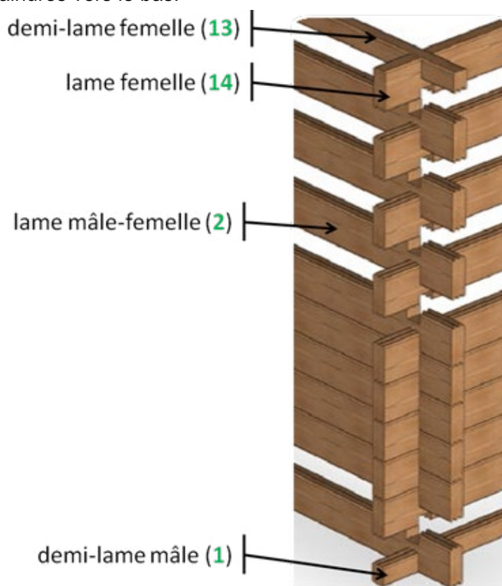
Figure 9 – Principe d'emboîtement des lames de bois
