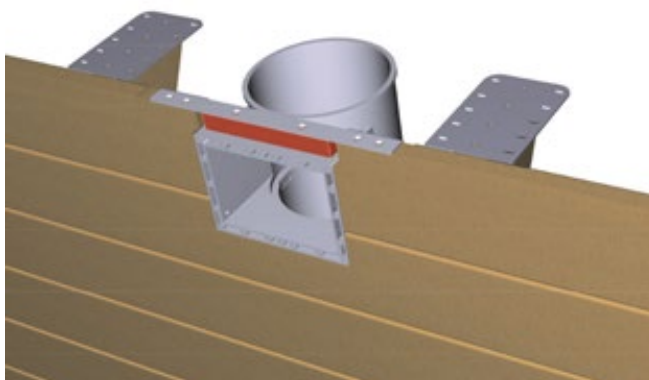
Figure 22 – Montage de l'équerre de skimmer
