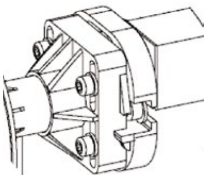
Figure 38 – Montage de l'axe sur le support de palier
