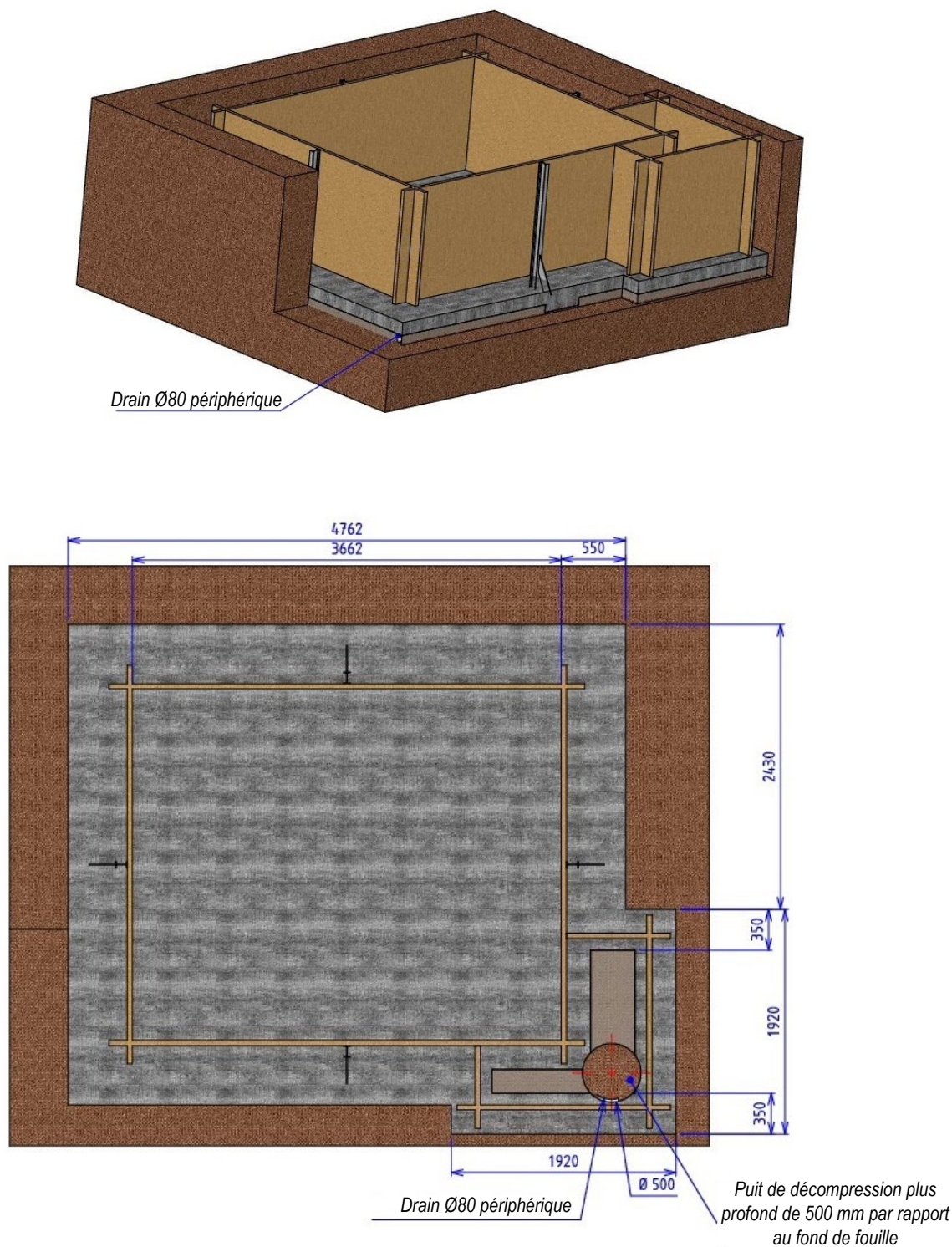
Figure 1 – Plan de pose du système de drainage
