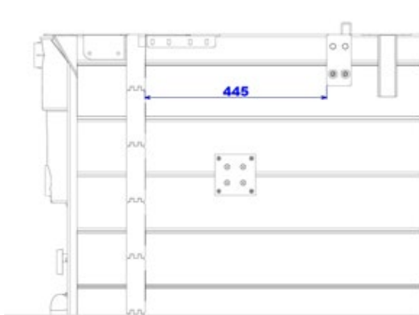
Figure 29 – Position de la contre-platine de support de poutre
