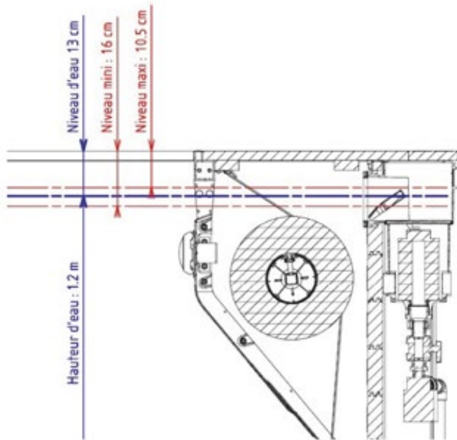
Figure 47 – Niveau d'eau dans le bassin
