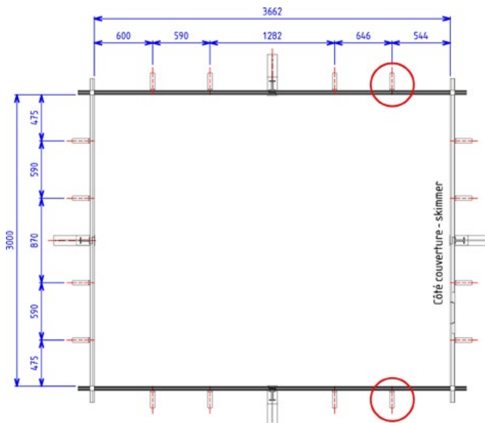
Figure 14 – Emplacement des consoles de margelles
