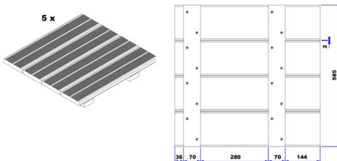
Figure 49 – Assemblage des caillebotis
