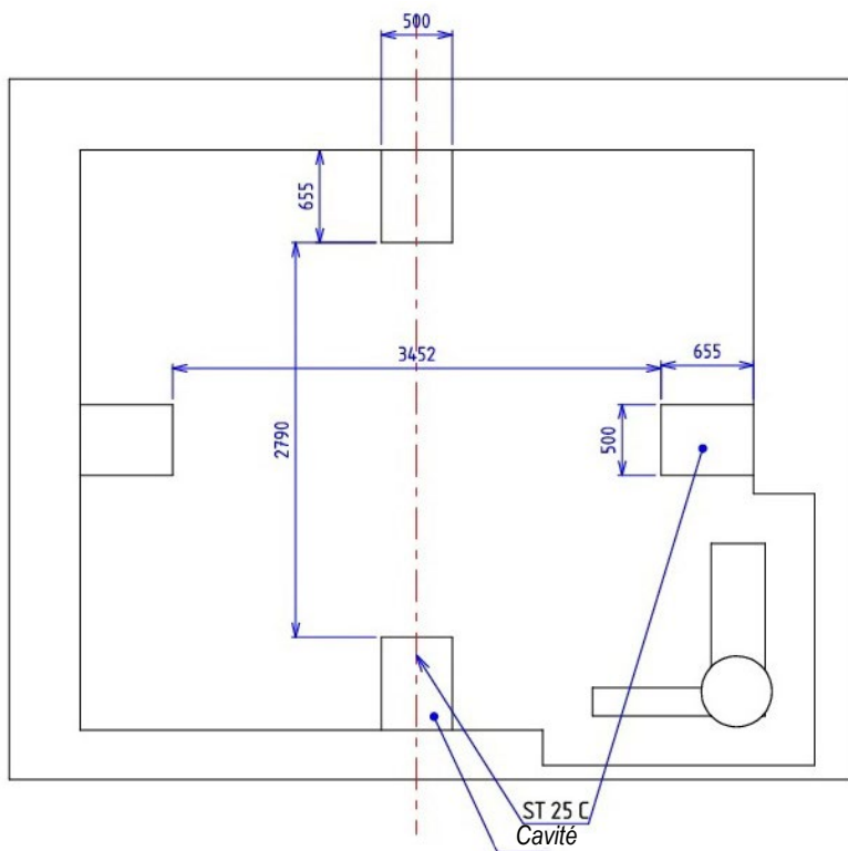
Figure 2 – Emplacements des cavités destinées à accueillir les jambes de force
