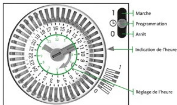
Figure 55 – Façade de l'horloge de filtration
