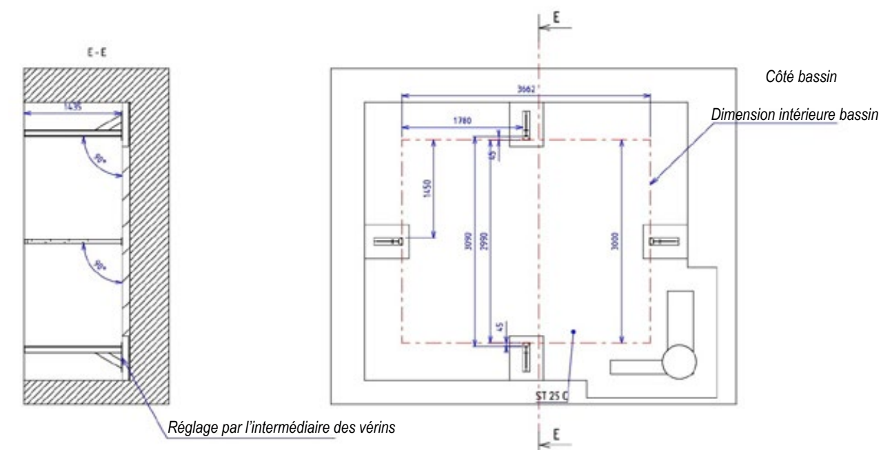
Figure 3 – a et b - Mise en place des vérins sur les jambes de force
