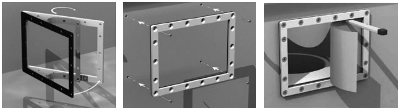
Figure 36 – Montage de la bride de skimmer
