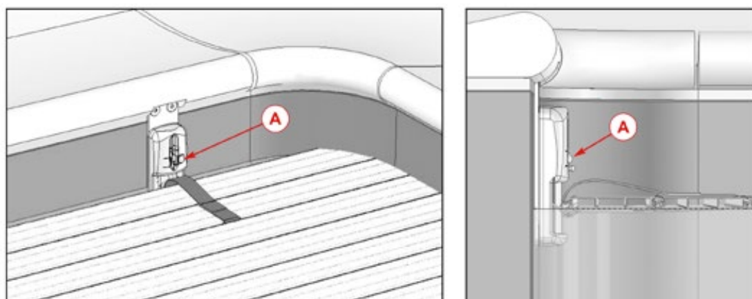
Figure 46 – Blocage et déblocage du tablier
