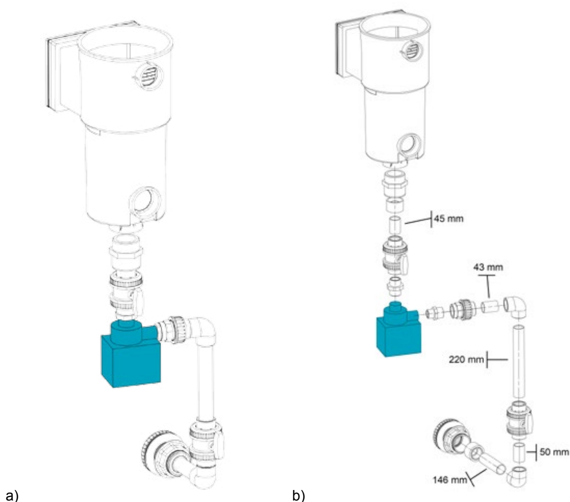
Figure 24 – a et b Tuyauterie pour la filtration
