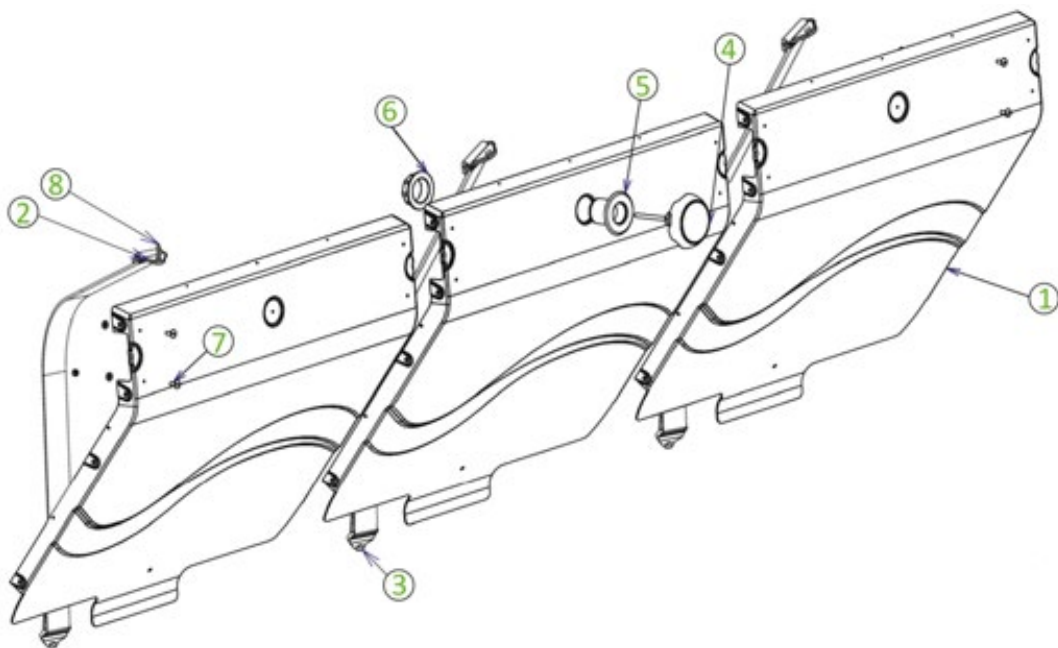
Figure 41 – Montage de la paroi de séparation et du projecteur
