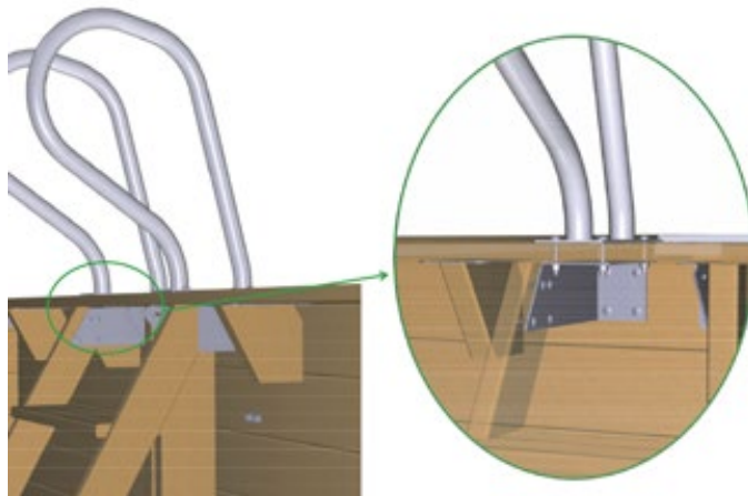
Figure 51 – Fixation des crosses d'échelle
