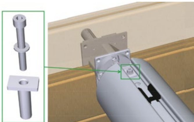
Figure 39 – Verrouillage de l'arbre dans l'axe de couverture automatique
