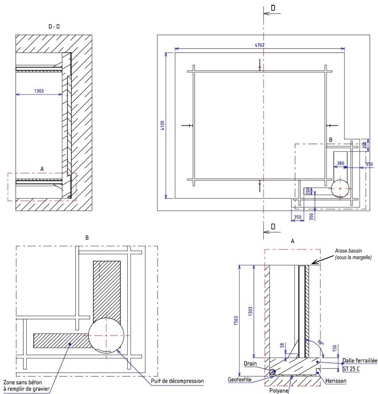
Figure 5 – Caractéristiques de la dalle de béton
