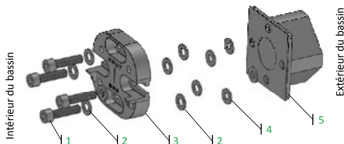
Figure 35 – Montage de la bride porte-palier
