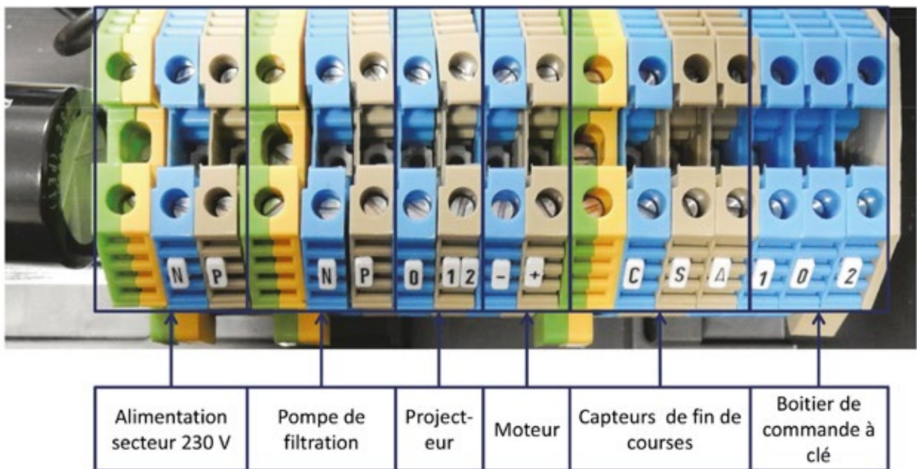
Figure 53 – Coffret électrique de la PISCINE URBAINE
