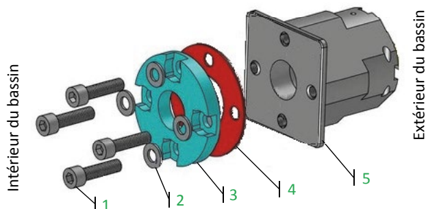
Figure 34 – Montage de la bride de traversée de paroi
