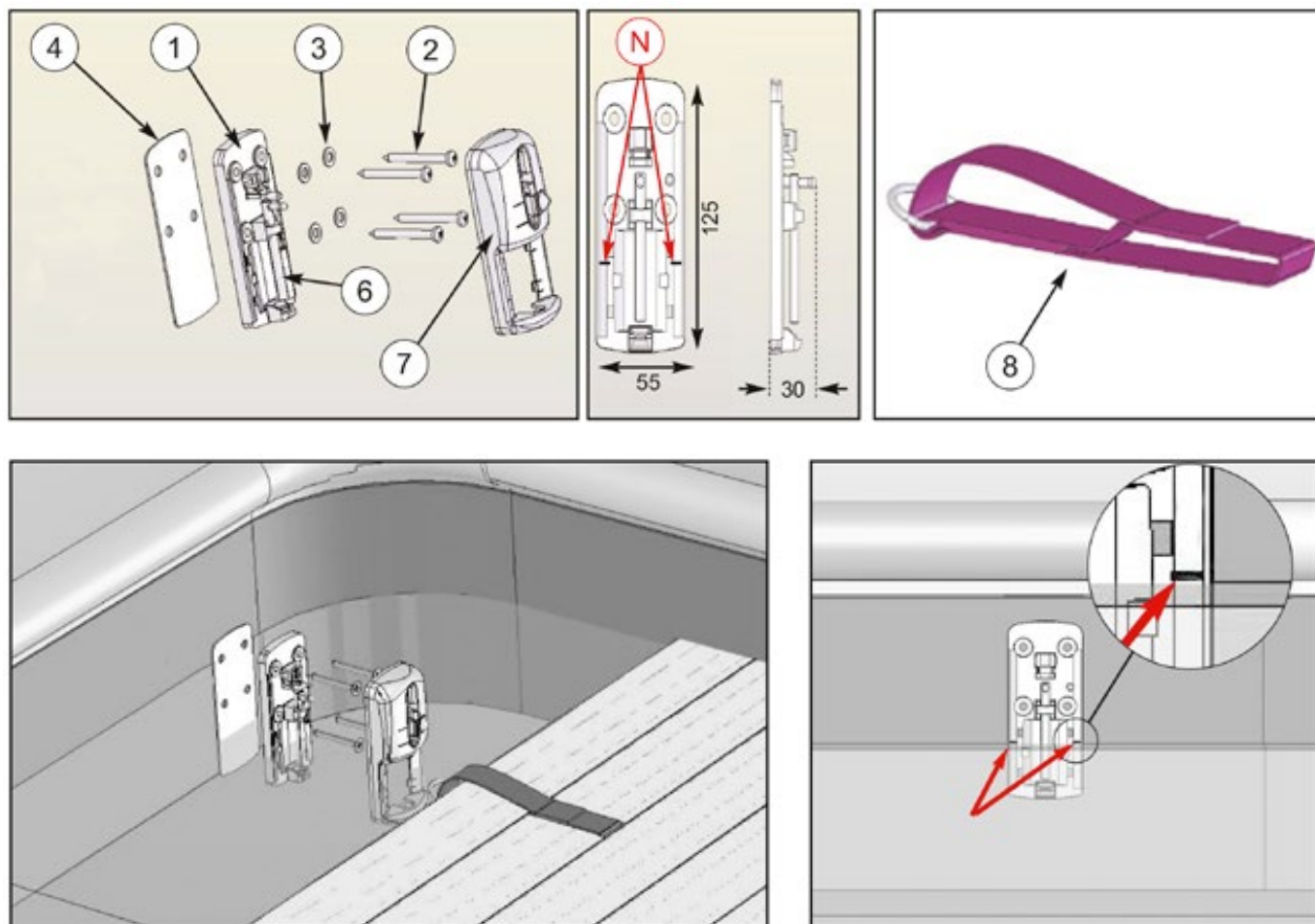
Figure 45 – Pose des accroches de tablier
