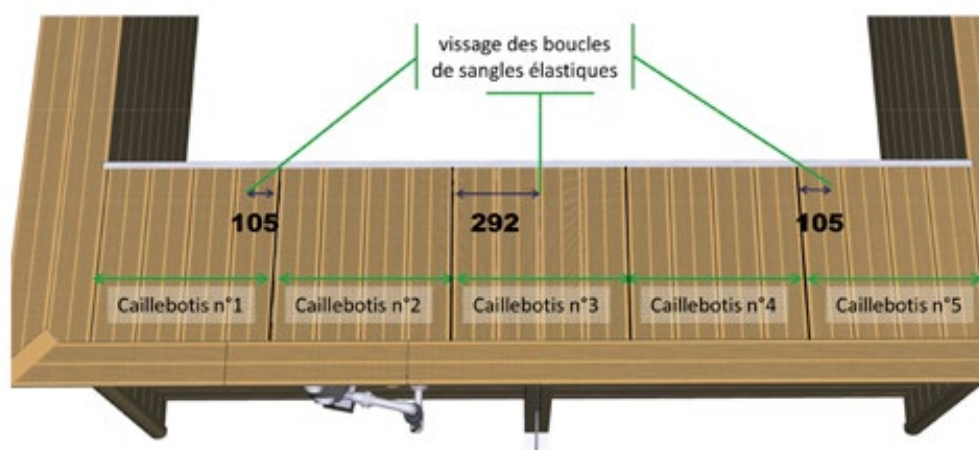
Figure 50 – Fixation des sangles élastiques sous les caillebotis
