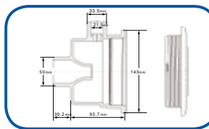
Côte SP1450TE
