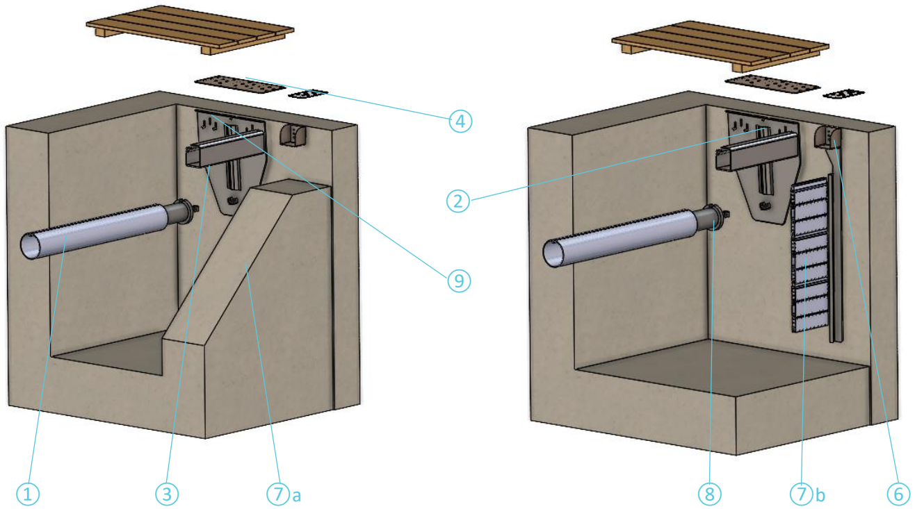
Exemple d'installation avec configuration sous margelle
