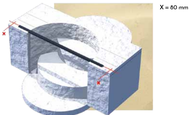
Schéma de placement du profil de remplacement des margelles
