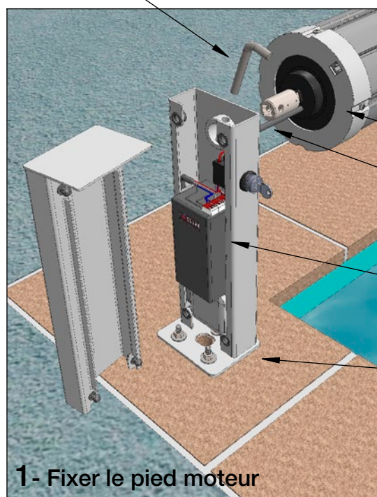
Goupille arbre moteur
